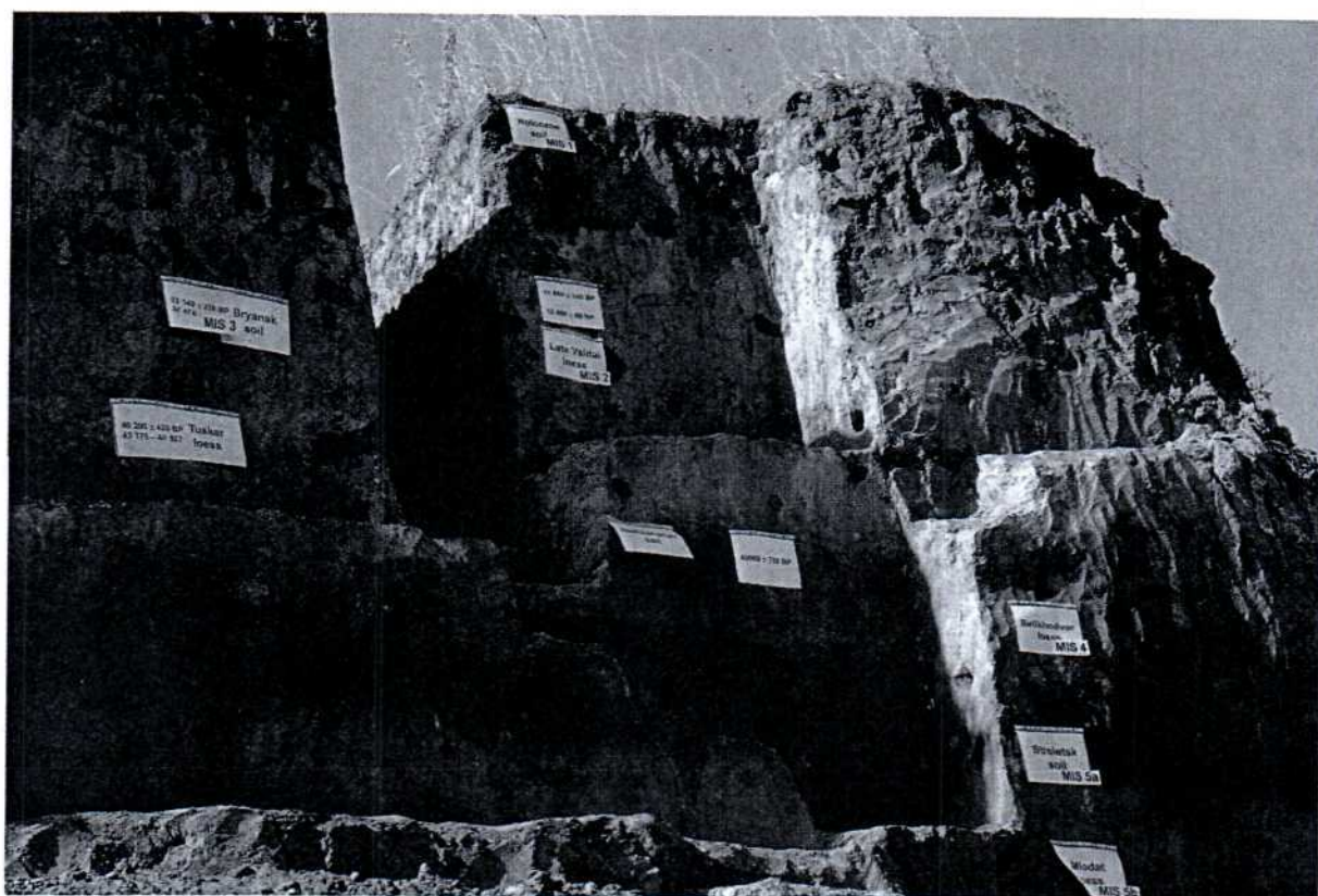
Фото 4. Почвенный профиль
